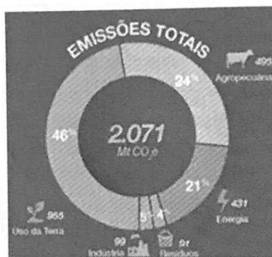
Figura 1.3a. Emissões de gases de efeito estufa por setor no Brasil em 2017 (Fonte: SEEG 2018)
