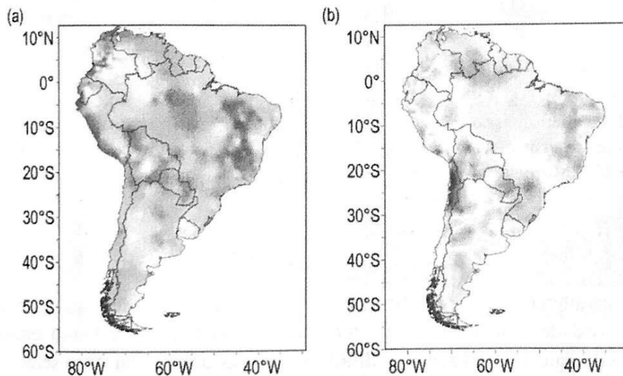
Figura 1.4. Aumento de temperatura já observado e mudanças na chuva já ocorridas na América do Sul no período 1981-2010 (BAMS, State of the climate 2015).
