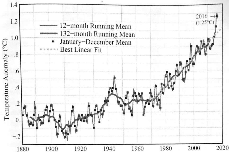
Figura 1.2. Temperatura média de nosso planeta de 1880 a 2016, mostrando o forte aumento, principalmente depois de 1970. O aumento médio global é de 1.25 grau Celsius em relação à média de 1850 a 1900. Algumas regiões brasileiras como o Nordeste já se aqueceram 1.6 grau Celsius. Fonte: GISS Surface Temperature Analysis (GISTEMP v. 3).
