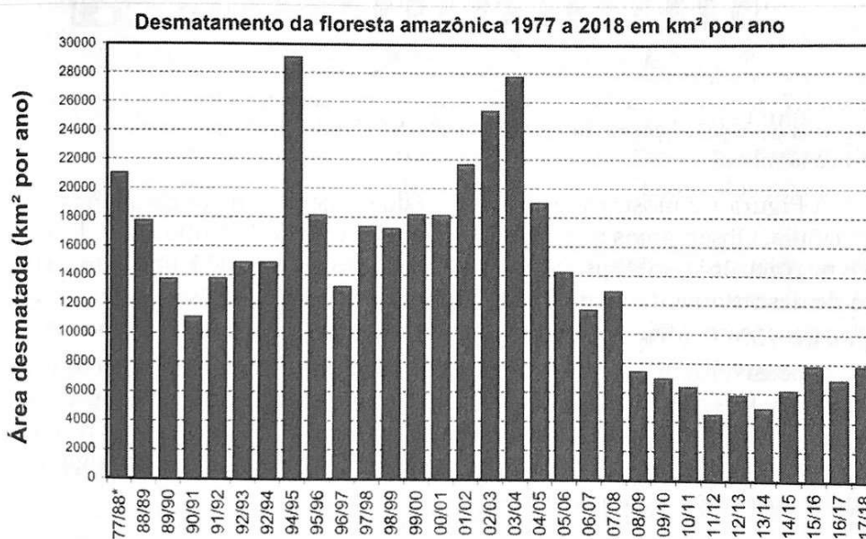
Figura 1.6. Taxas de desmatamento anual da floresta amazônica de 1977 a 2018. Fonte: INPE/PRODES.
