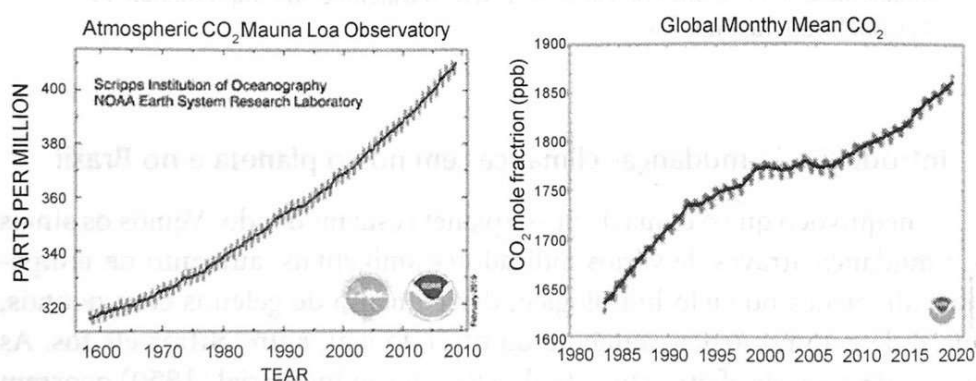
Figura 1.1. Concentração atmosférica de CO 2 de 1960 a 2018, mostrando o forte aumento da concentração de gases de efeito estufa na atmosfera. A figura à direita mostra a concentração de metano de 1984 a 2018, também com forte aumento na concentração.
