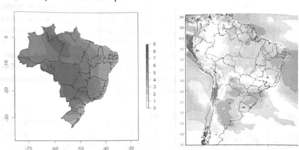
Figura 1.5. Observamos no gráfico à esquerda o aumento previsto de temperatura no cenário RCP 8.5 (equivalente a manter as taxas de emissões crescentes como atualmente) para o período de 2071 a 2099, comparado a valores pré-industriais (antes de 1850). A figura à direita mostra as alterações na taxa de precipitação, com valores decrescentes em marrom e aumentos em azul. Simulações climáticas realizadas pelo INPE.
